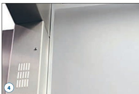
Löstagbar karm, automattörr för enkel service av låsbana
